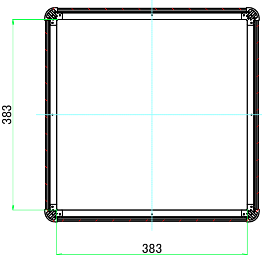
C-C ( 1 : 7.5 )
