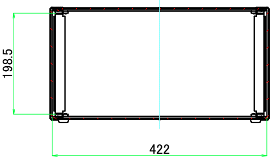
B-B ( 1 : 7.5 )
